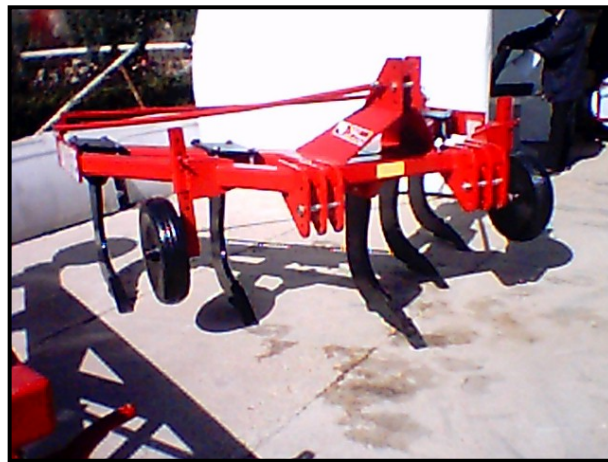
شکل ۴- زیرشکن ۵ شاخه با قاب V شکل و شاخه‌های C شکل
